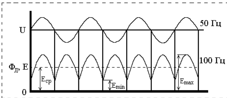
Рисунок 1. Зависимость светового потока от напряжения питания
