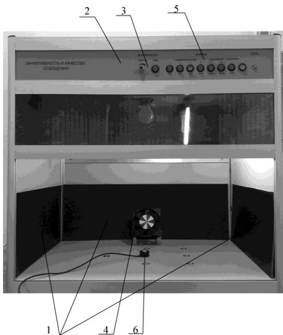
Рисунок 2. Схема лабораторной установки
