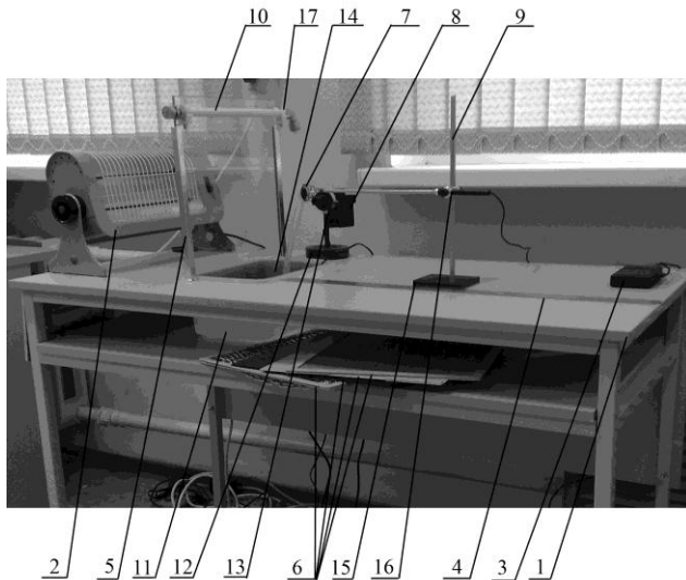
Рис. 1. Внешний вид установки
