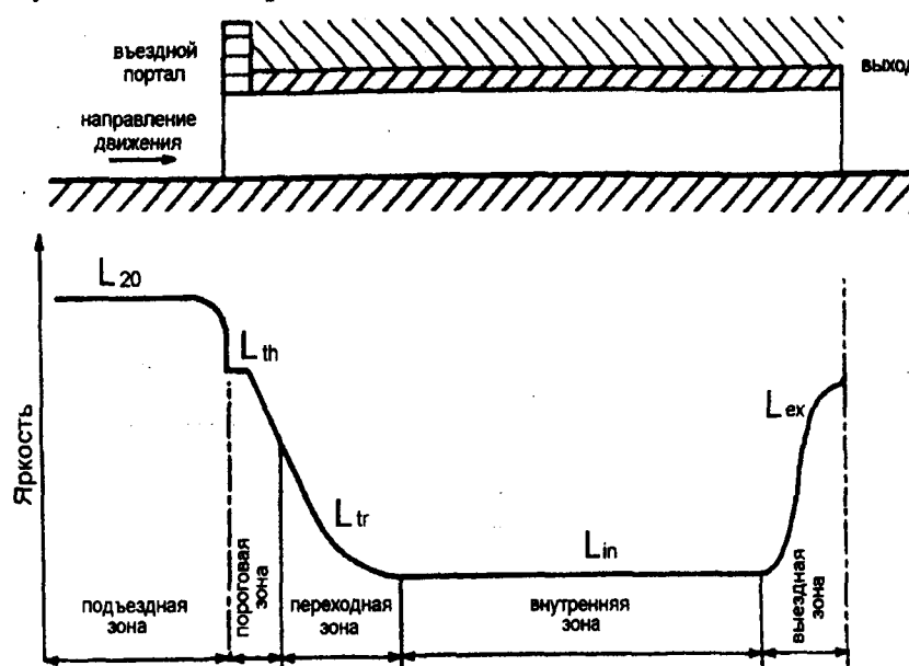
Рисунок Ж.1 — Яркостные зоны тоннеля в дневном режиме
