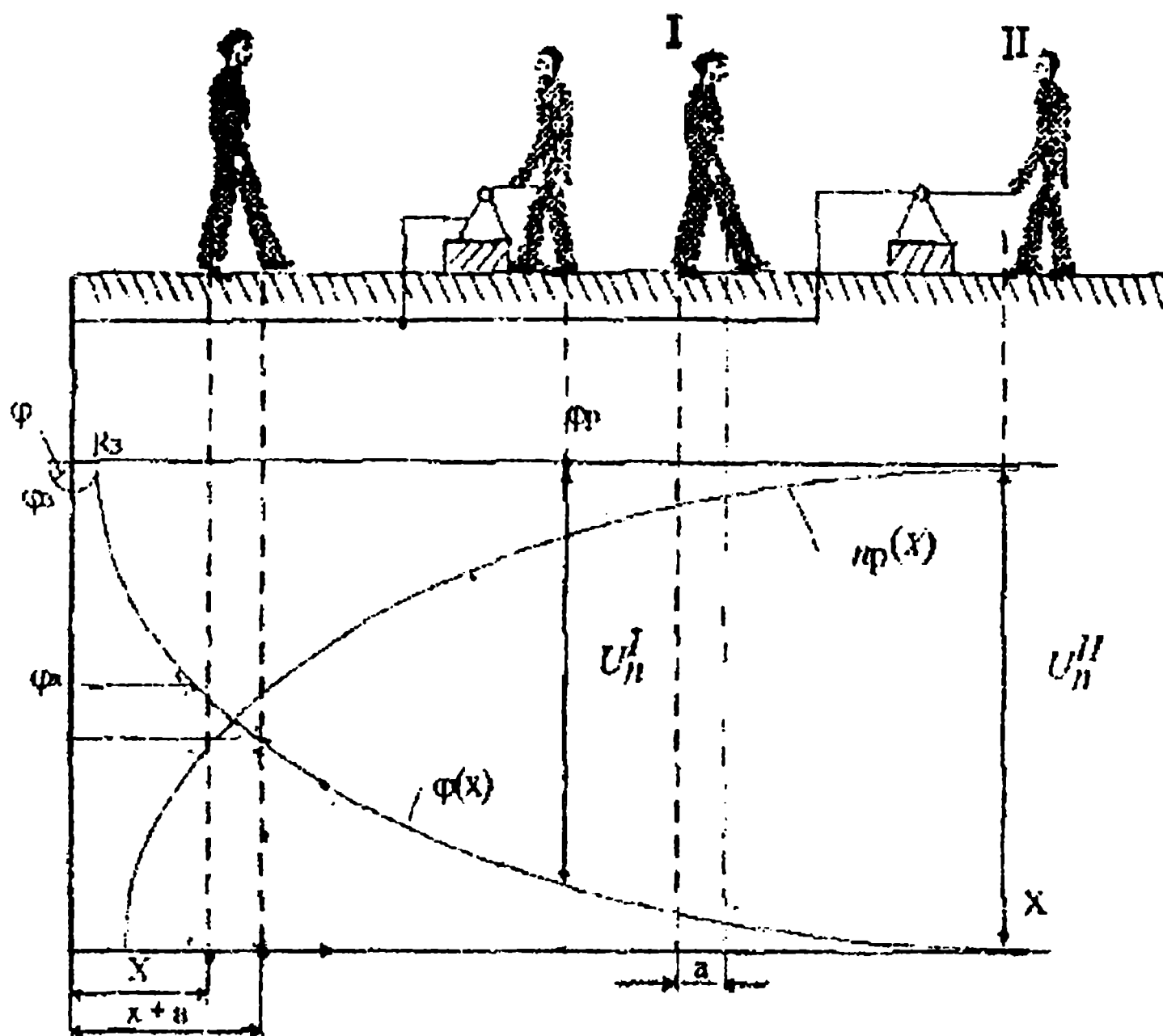
Рис.1. Явление растекания тока в земле
